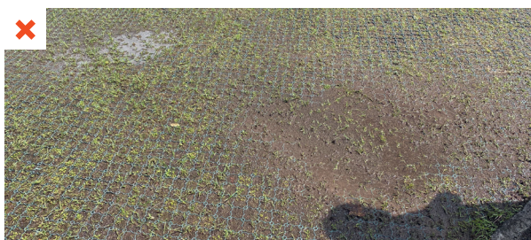
Disparition de la végétation mise en place du fait d'un défaut de drainage et d'un écrasement de la végétation par les véhicules dû. Le remplissage des alvéoles est trop important. ©AQC
