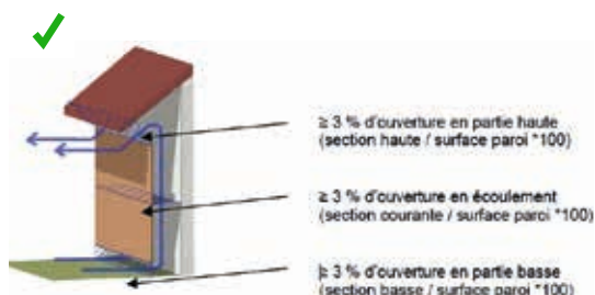
Figure 2 : pare-soleil ventilé (cf. annexe III – 3.3.2' de l'arrêté du 17 avril 2009)
